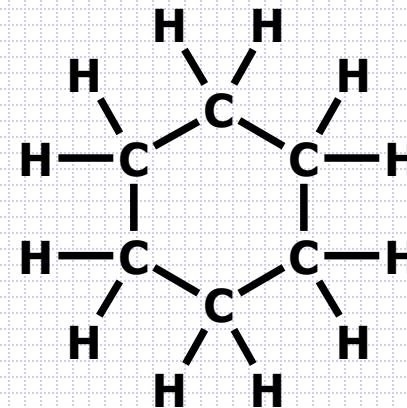
Cyclohexan
